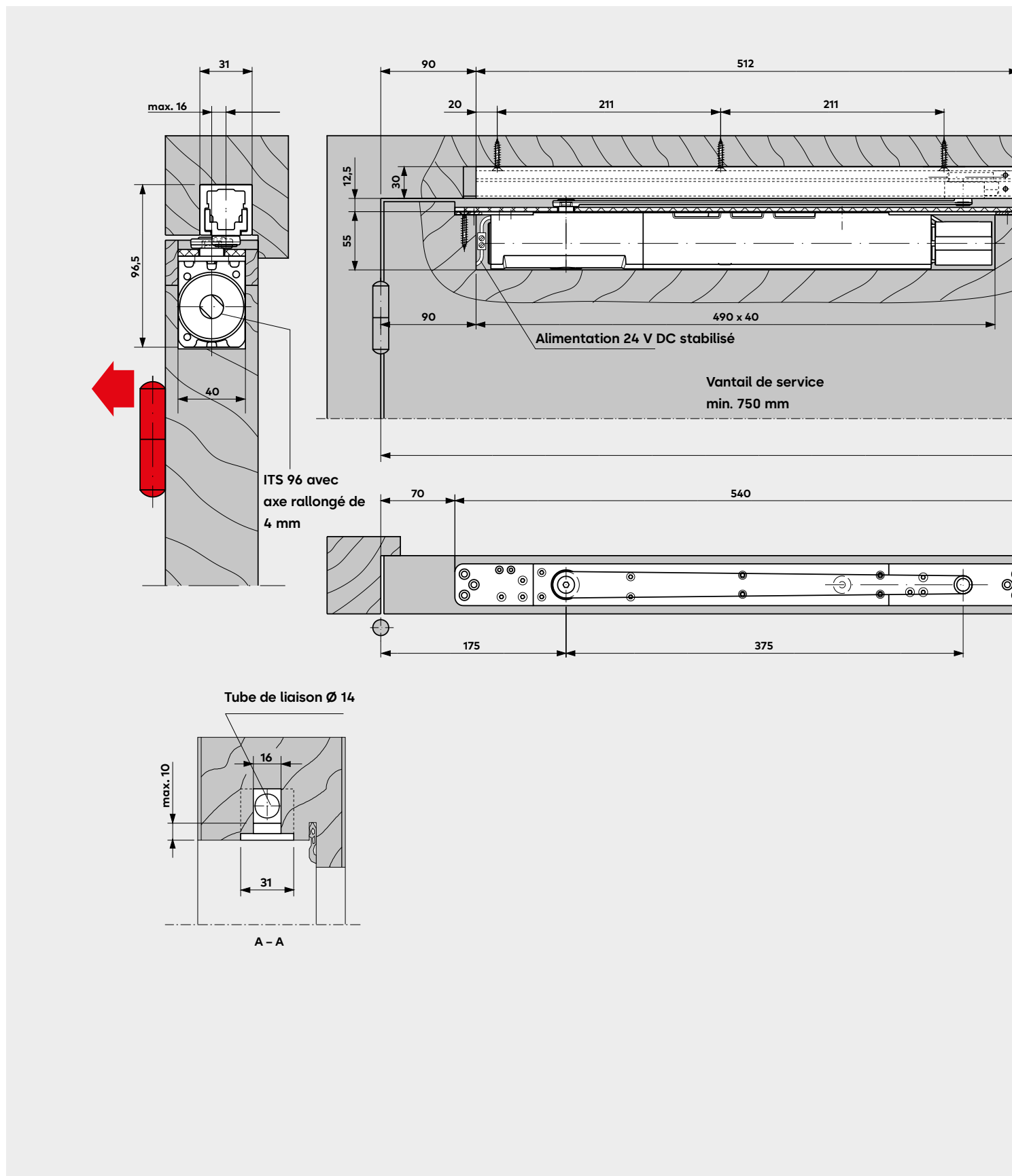
Ferme-porte ITS 96 FL dans le vantail de service et ITS 96 dans le vantail semi-fixe avec glissière G 96 GSR Exemple vantail de service DIN-L. Sur vantail DIN-R, le schéma serait symétrique
