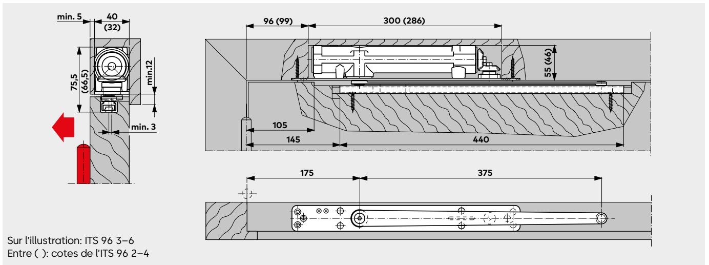
Ferme-porte ITS 96 avec glissière G 96 N20 dans une porte bois en montage renversé Exemple sur porte DIN-L. Sur porte DIN-R, les schémas seraient symétriques
