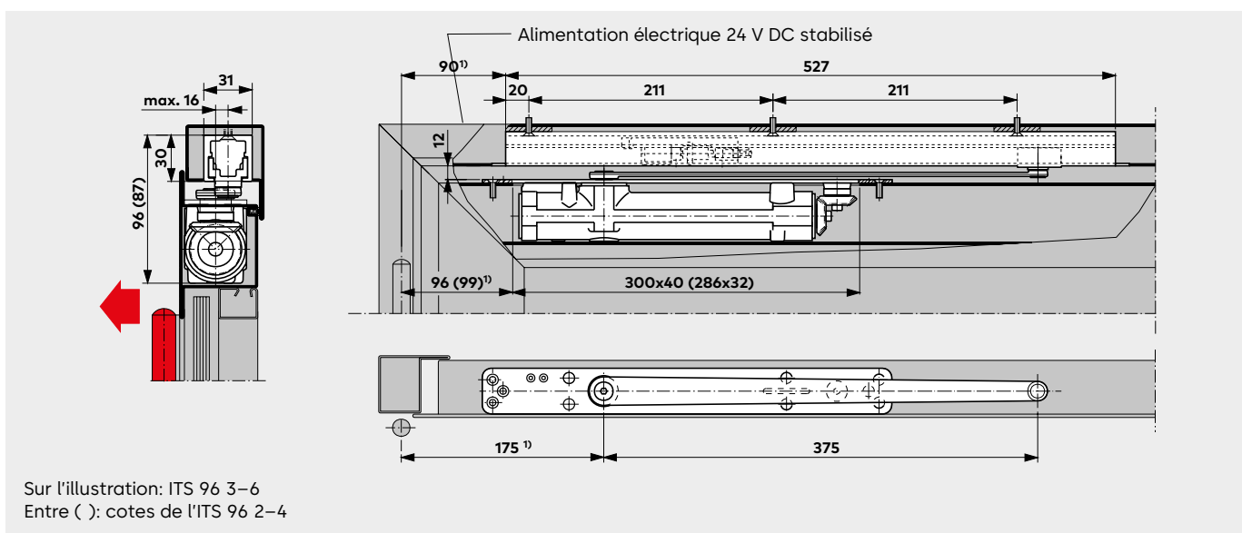
Ferme-porte ITS 96 avec glissière G 96 EMF dans une porte en profilé Exemple sur porte DIN-L. Sur porte DIN-R, les schémas seraient symétriques 1) construction en profilé avec équerre + 25 mm
