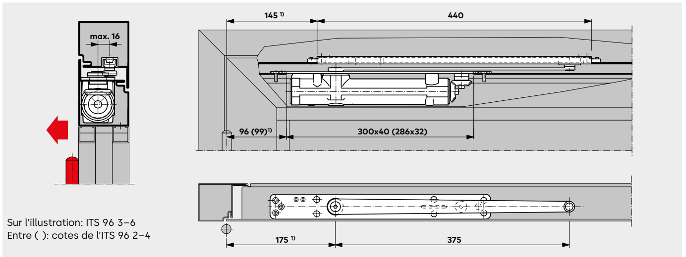
Ferme-porte ITS 96 avec glissière G 96 N20 dans une porte en profilé Exemple sur porte DIN-L. Sur porte DIN-R, les schémas seraient symétriques. 1) construction en profilé avec équerre + 25 mm
