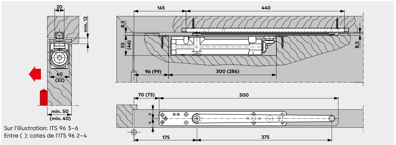
Ferme-porte ITS 96 avec glissière G 96 N20 dans une porte en bois Exemple sur porte DIN-L. Sur porte DIN-R, les schémas seraient symétriques
