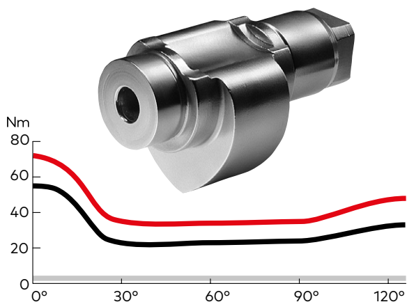
Courbes des moments d'un ferme-porte à glissière ITS 96 force 3-6 EN, réglé au maximum
