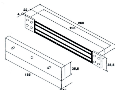
IGEM 2-35,5 schéma
