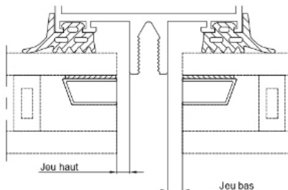
Figure 13 - Jeux mini/maxi entre meneau/traverse et remplissage
