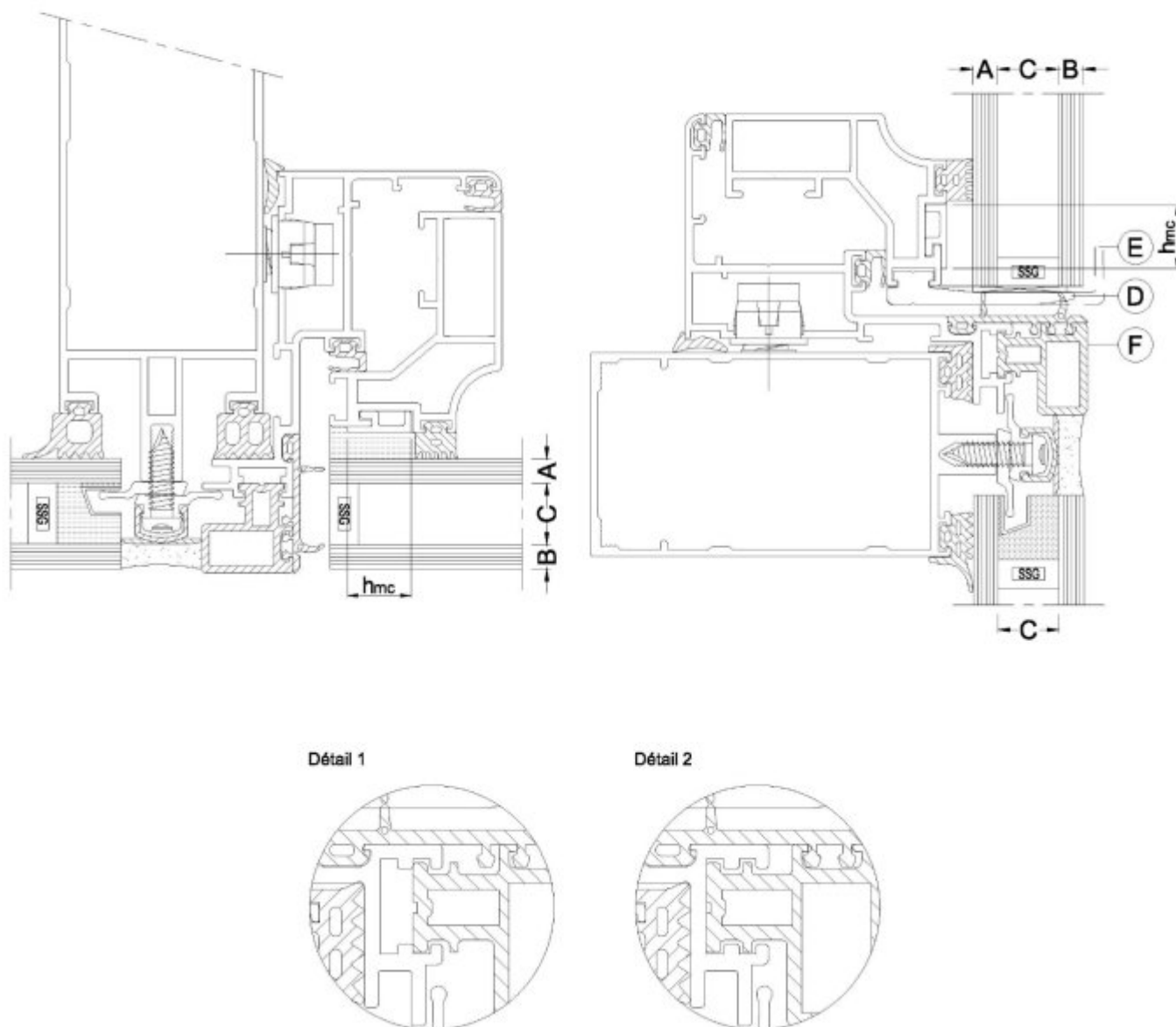
Figure 29 - Coupes de principe sur ouvrant vers l'extérieur - Vitrage à bord décalé
