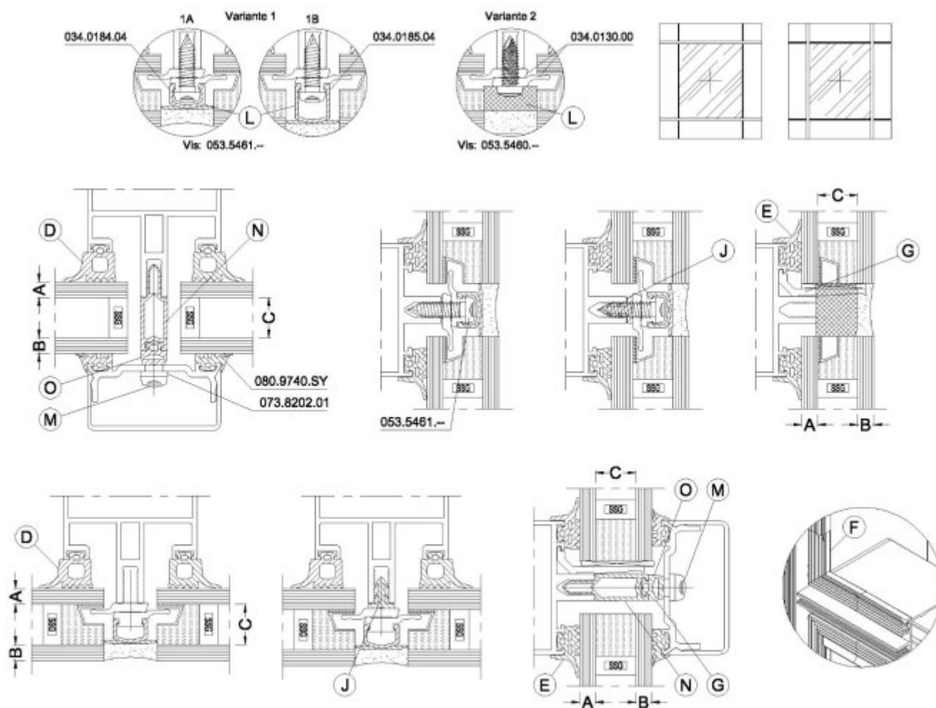
Figure 25 - Partie fixe - Tableau de vitrage – Détails du panneau ventilé
