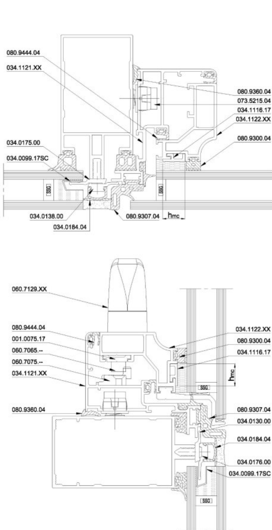
Figure 31 - Tableau de vitrage pour ouvrant vers l'extérieur - Vitrage à bord décalé
