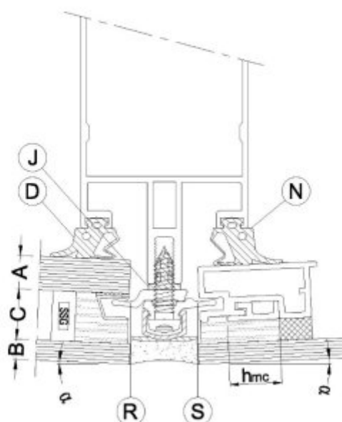
Figure 36 - Tableau de vitrage pour solutions d'angle - 2.5° - 5° - 7.5° - A côté d'un ouvrant
